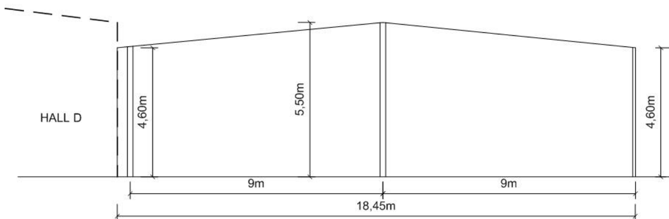
COUPE HALL E éch: 1/100
